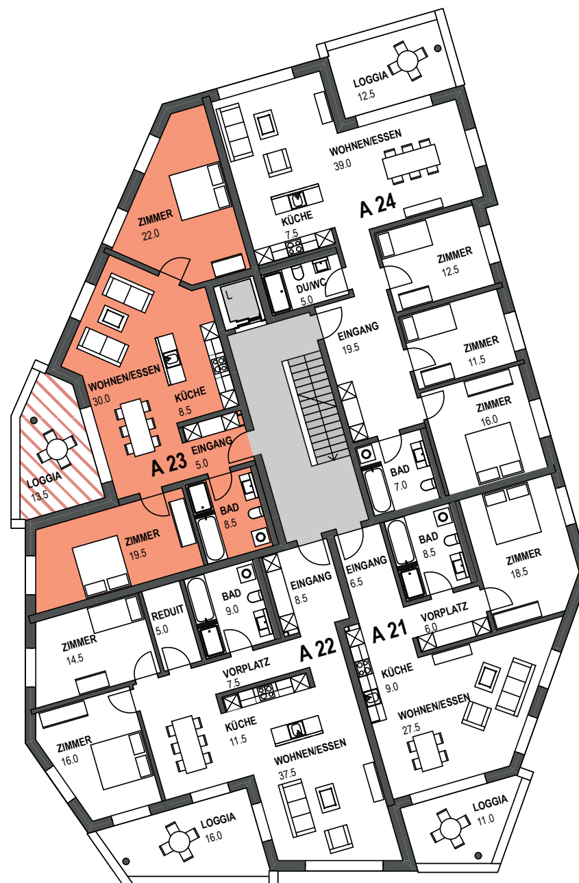
Grundriss 1. Obergeschoss Haus A
